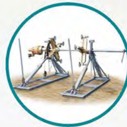
Alzabobina CVI602 Alzabobina Hidráulico hasta 6 Tn.
